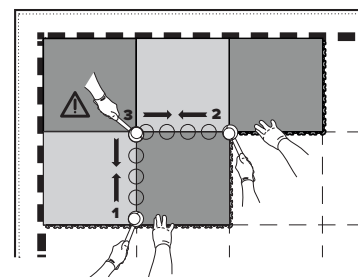
Rys. nr 4 Sposób układania płytek INVISIBLE, BUSINESS
