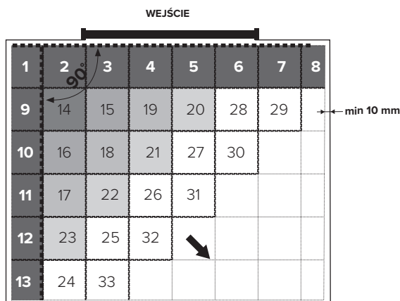
Rys. nr 2 Układanie Fortelock INVISIBLE, BUSINESS
