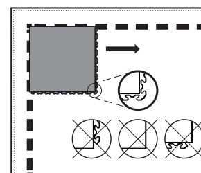
Rys. nr 3 Kierunek układania płytek INVISIBLE, BUSINESS
